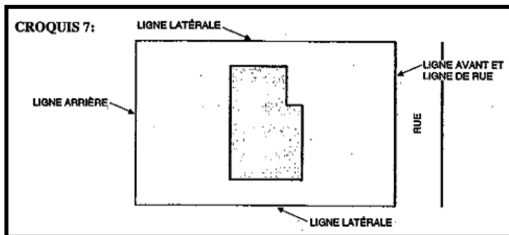
CROQUIS 7. Type de ligne constituant un lot
