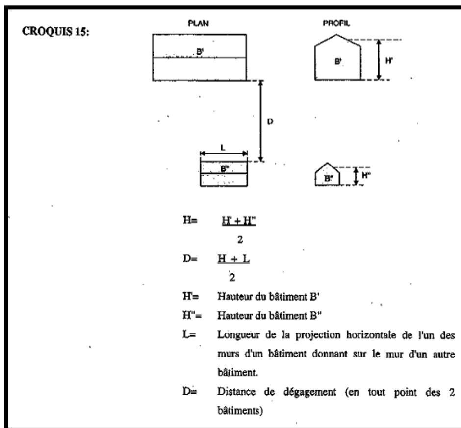
CROQUIS 15. Calcul de la distance de dégagement des bâtiments complémentaires par rapport aux bâtiments principaux dans les zones à dominance autre que résidentielle
