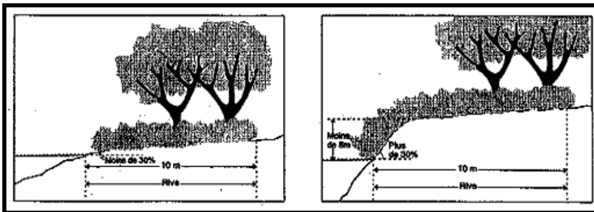
CROQUIS 10a. Coupe transversale illustrant une pente inférieure à 30%
