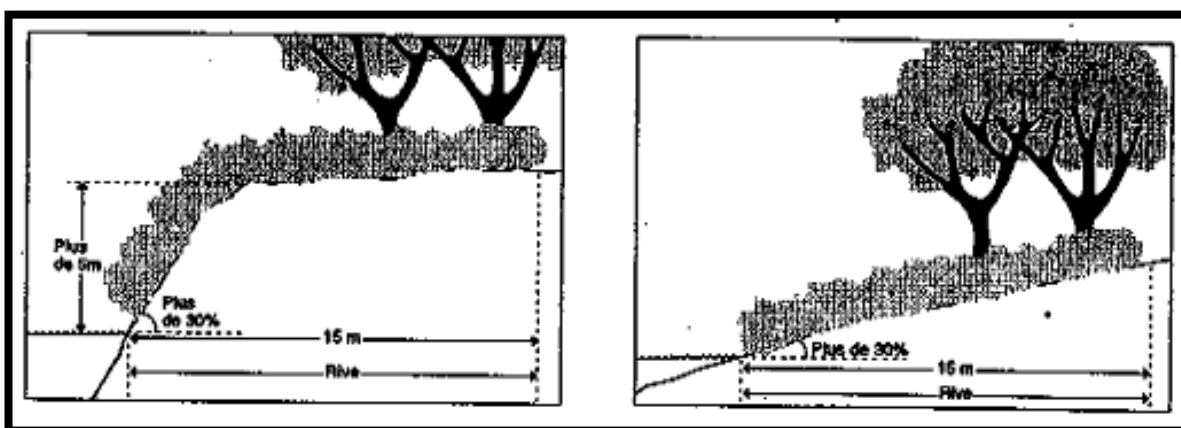
CROQUIS 10b. Coupe transversale illustrant une pente supérieure à 30%
