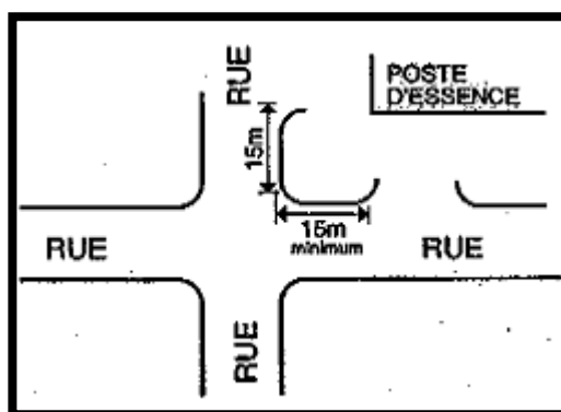
CROQUIS 23. Distance minimale à respecter entre une allée d'accès et une intersection
