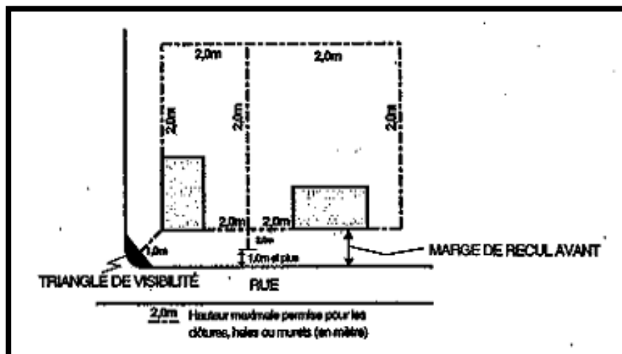
CROQUIS 16. Hauteur des clôtures permises en fonction de leur localisation sur le terrain
