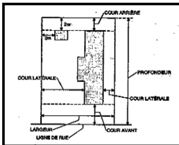
CROQUIS 24. Implantation perpendiculaire à la rue d'une maison unimodulaire
