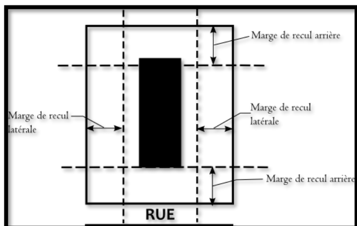
CROQUIS 21. Implantation d'un bâtiment prohibé après le déplacement
