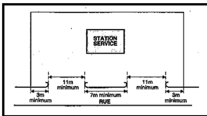
CROQUIS 22. Normes à respecter dans l'aménagement des allées d'accès à une station-service
