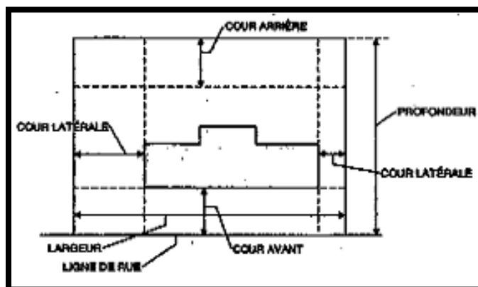
CROQUIS 25. Implantation perpendiculaire d'une maison unimodulaire
