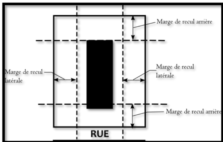
CROQUIS 20. Implantation d'un bâtiment autorisé après le déplacement
